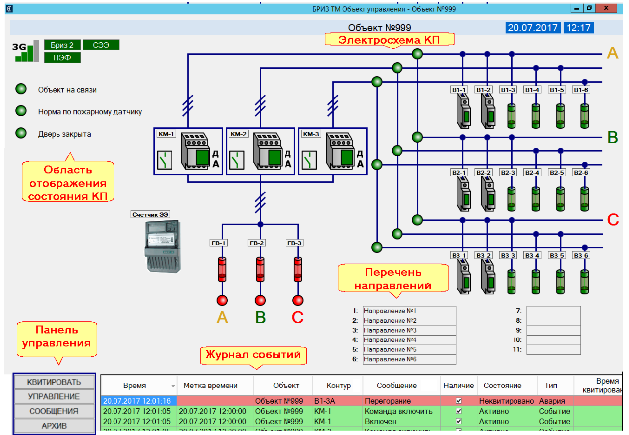
Рисунок 7 - Мнемосхема КП
