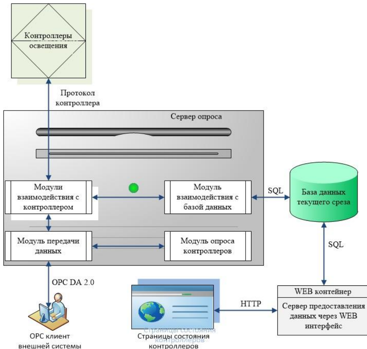
Рисунок 9 - Функциональная схема сервера АСУО «БРИЗ»
