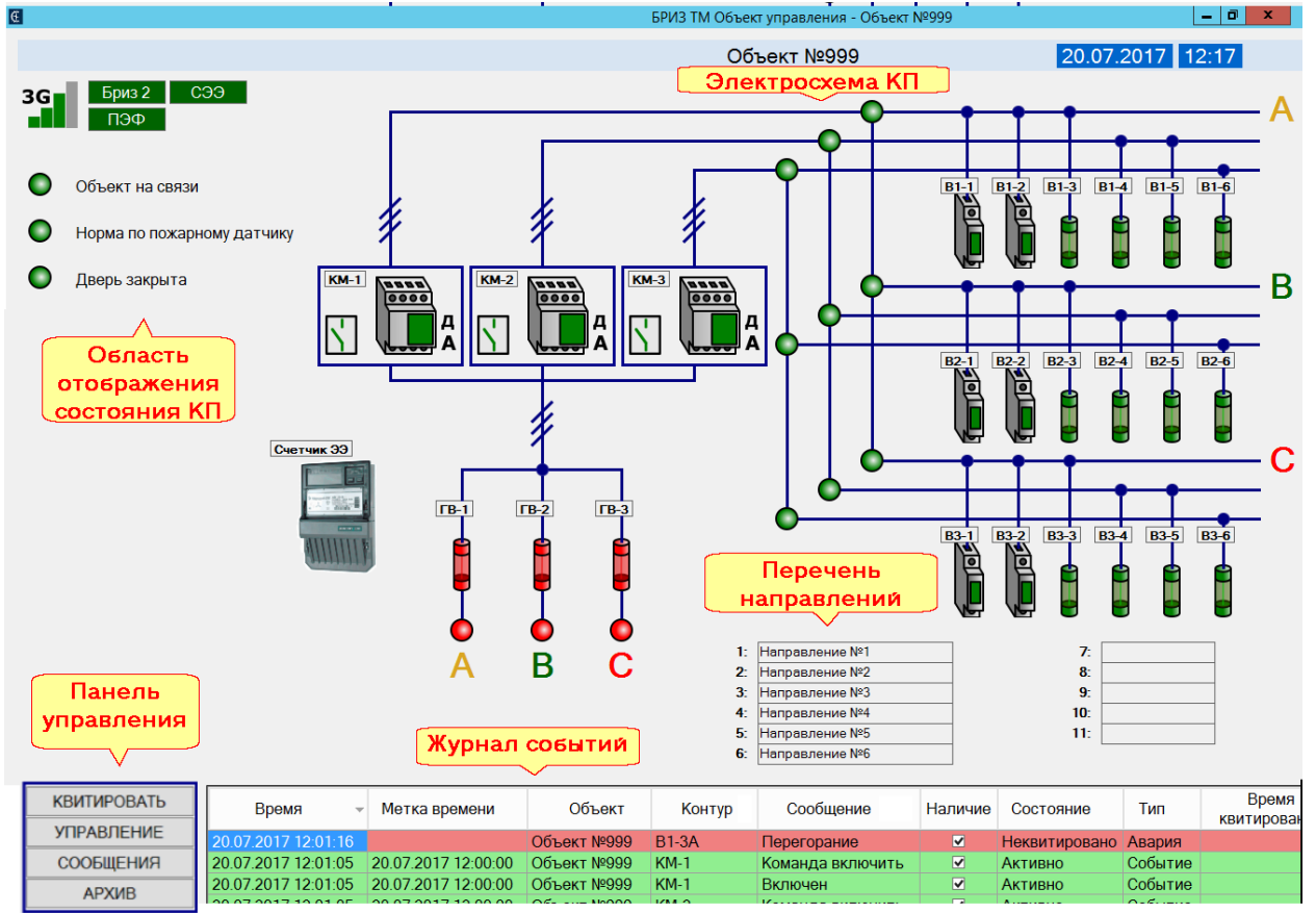
Рисунок 7 - Мнемосхема КП
