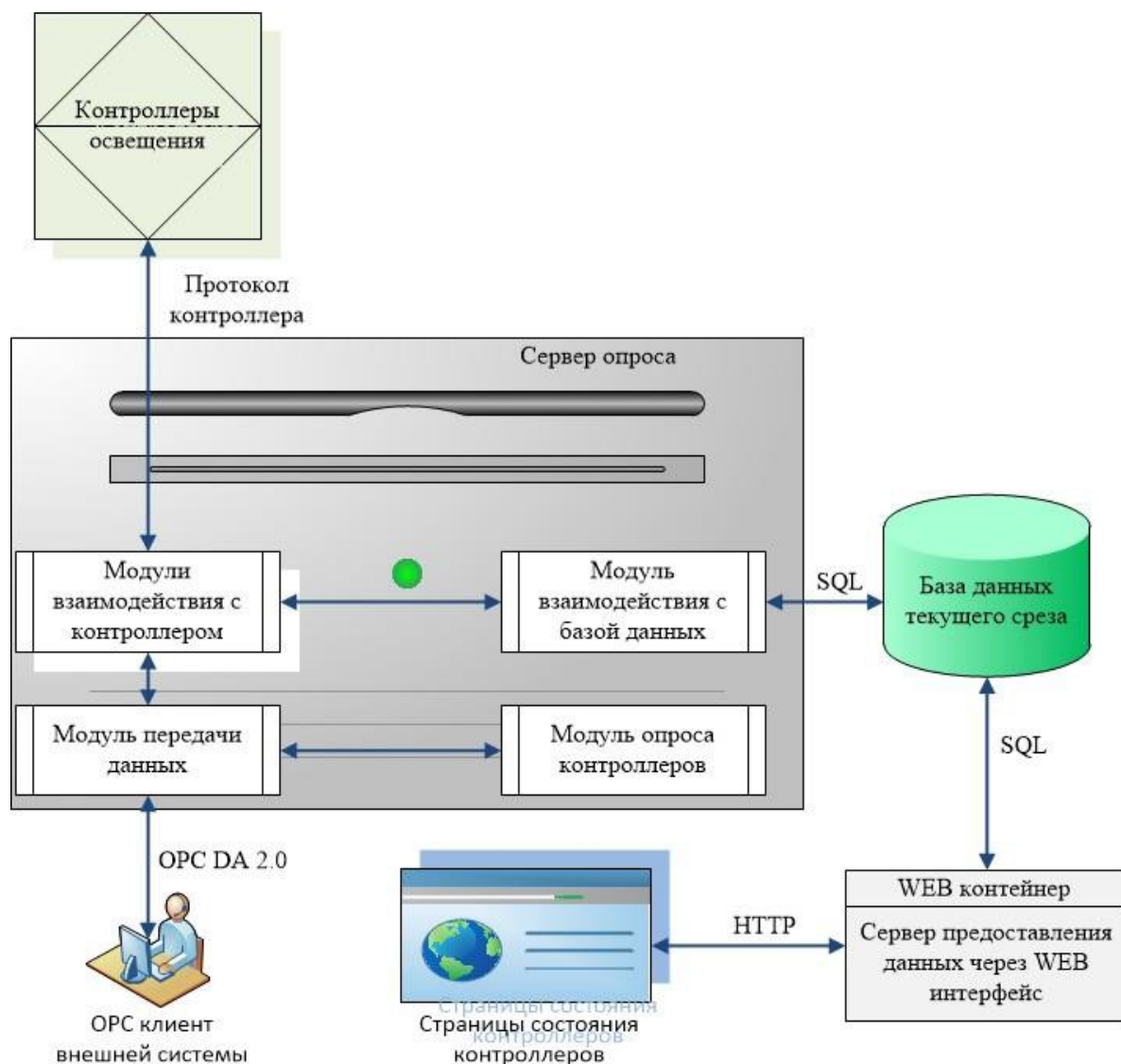
Рисунок 9 - Функциональная схема сервера АСУ «БРИЗ»
